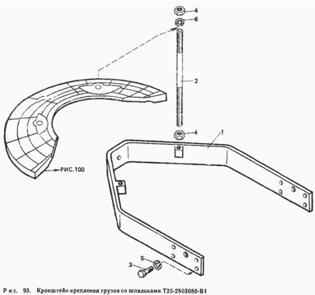
Рис. 093. Кронштейн крепления грузов со шпильками Т25-2803080-В1.
